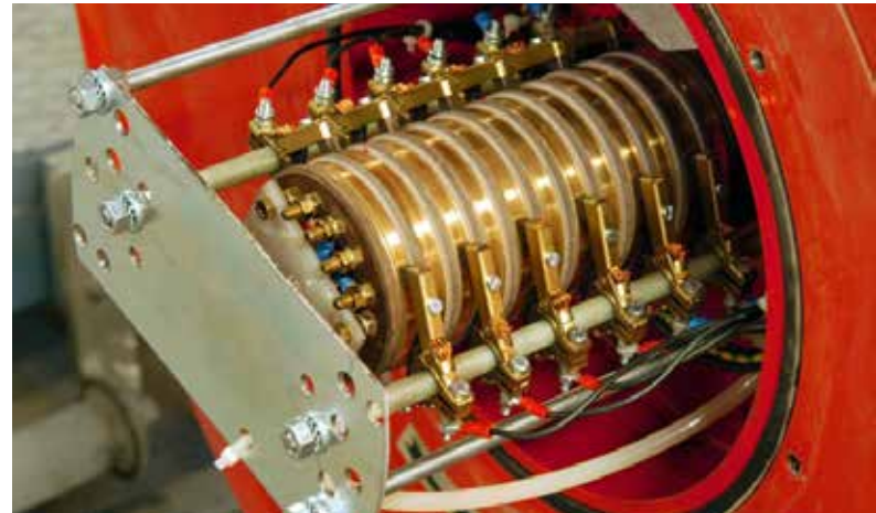
Endüstride Teknik Çözümler TAMBUR ENERJİ AKTARIM KOLLEKTÖRÜ (10A./40A. 3/16 kutuplu çeşitlerimizdir.)
